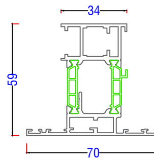
U44105 - Vent
