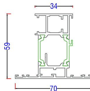
AL UK AW620 - Vent
