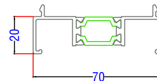
AL UK AW724 - Frame Extender
