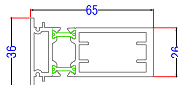
AL UK AW706 - Coupling Bar
