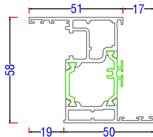
AL UK AW621 - Vent
